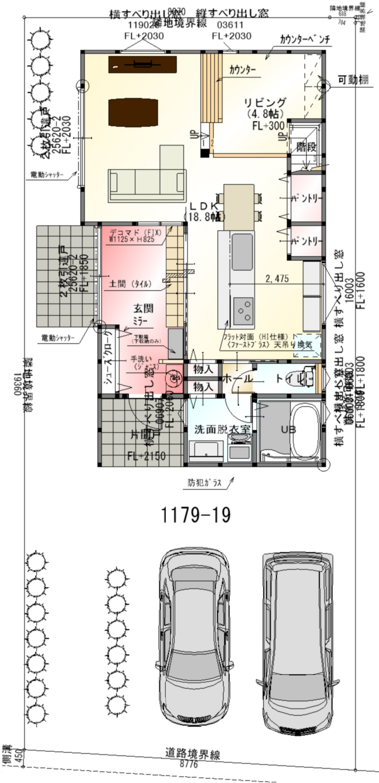
■ 1F PLAN
